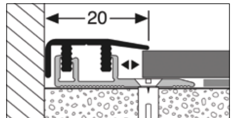
Clic-Endprofil Farben: Edelstahl, Bronze, Sand Längen: 1.000 mm, 2.700 mm
