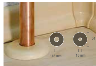
Heizrohrrosetten
