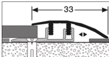
Clic-Ausgleichsprofil Farben: Edelstahl, Bronze, Sand Längen: 1.000 mm, 2.700 mm
