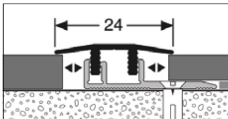
Clic-Übergangsprofil Farben: Edelstahl, Bronze, Sand Längen: 1.000 mm, 2.700 mm
